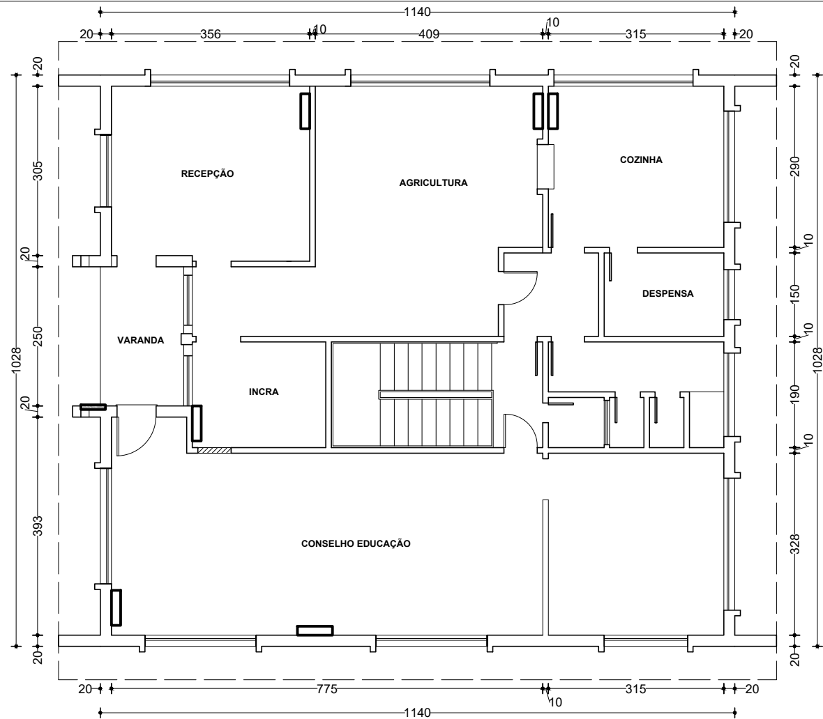
PLANTA BAIXA TÉRREO Área: 108,30m 2
